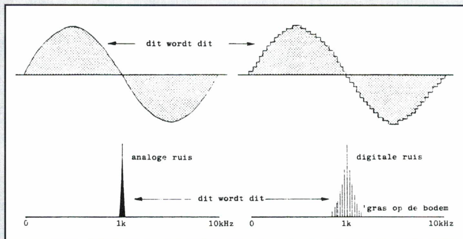
Fig. 2. Bij bandopnamen ontstaat een zekere mate van modulatie-ruis. Bij het digitale signaal met zijn vele spanningssprongen gaat dat nog wat verder en er is dan sprake van kwantiseringruis, die de klank enigszins rauw maakt.
